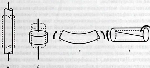
Рис. 9.1. Схемы деформации при разных способах нагружения. а — растяжение; б — сжатие; в — изгиб; г — кручение (стрелками показано направление нагрузки, пунктиром — начальная форма образцов).
