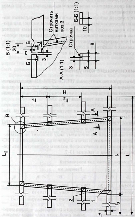
Рис. 13-1. Большая повязка для конечностей. 1 — полотнище; 2 — фиксирующая тесьма; 3 — строчка нитками; L — длина полотнища повязки с тесьмами; L_2 — длина узкой части полотнища повязки; L_1 — длина широкой части полотнища повязки; I_3 — длина фиксирующей тесьмы; I_4 — ширина фиксирующей тесьмы; N — ширина всей повязки; h_1 — расстояние между первой и второй тесьмами (отсчёт от узкой части повязки); h_2 — расстояние между второй и третьей тесьмами повязки.
