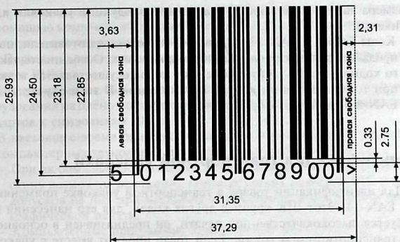
Рис. 6-1. Содержание штрихового кода EAN-13.
